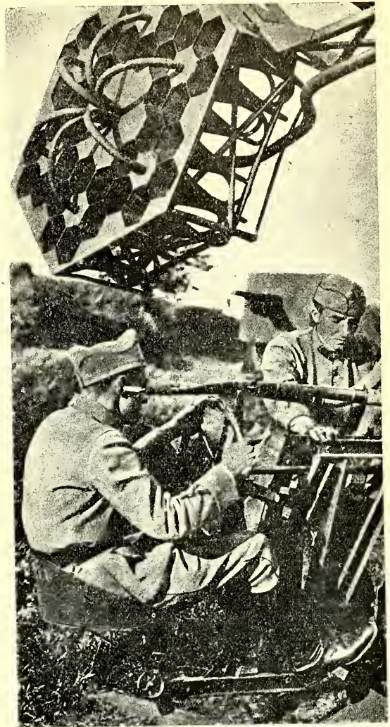
Звукоулавливающий аппаратъ, вновь принятый въ войскахъ воздушной обороны,
